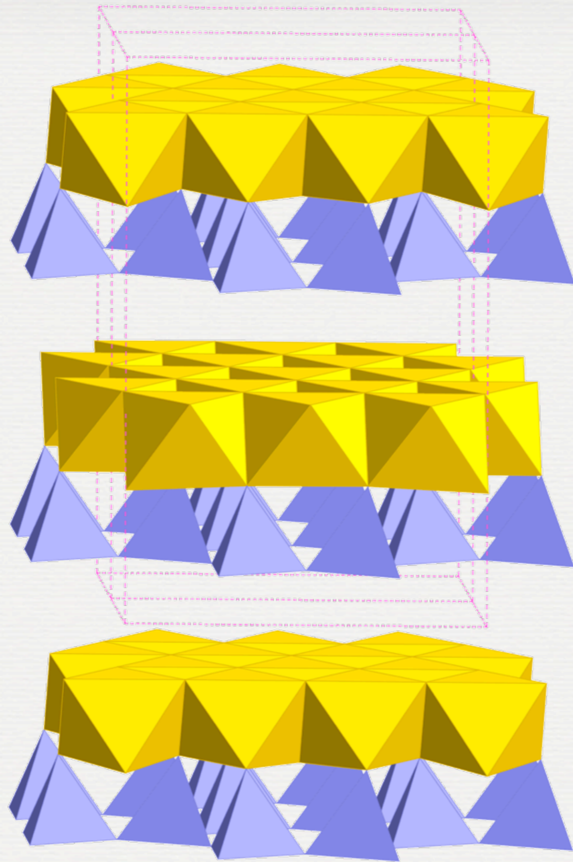
Antigorite
