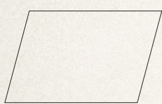
p1
