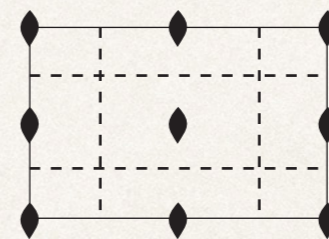
p2gg
