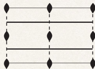
p2mg
