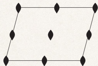
p2
