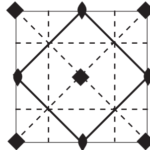
p4gm
