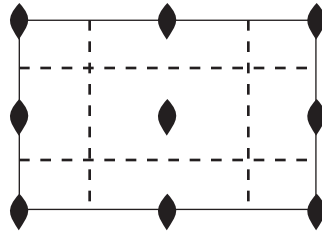
p2gg
