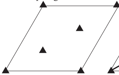
p3
