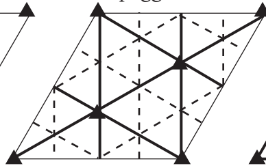
p3m1
