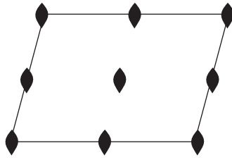
p2
